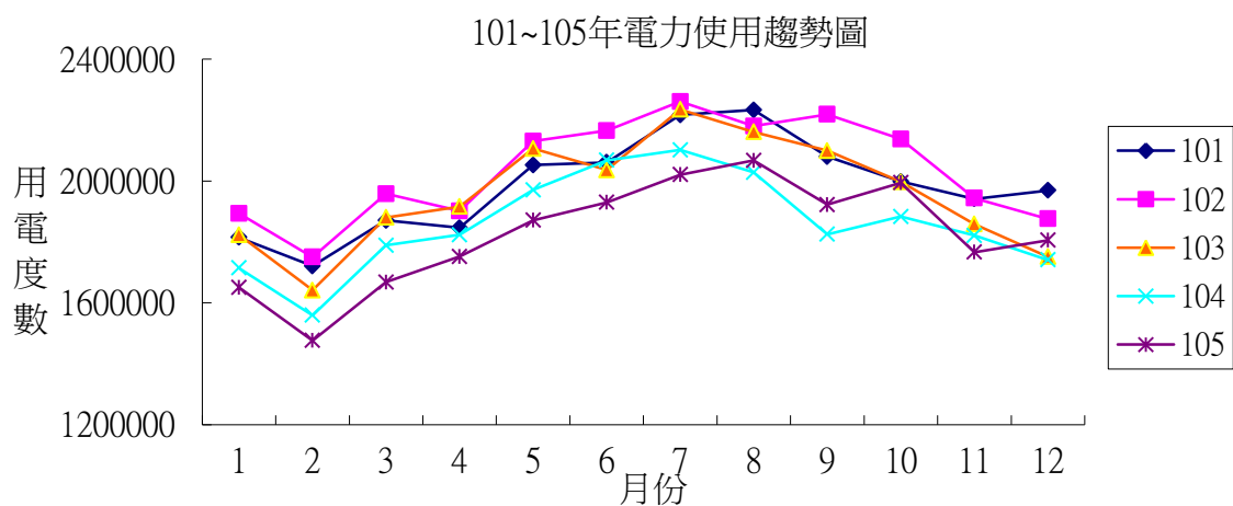
台北晶華酒店近五年能源使用趨勢圖
